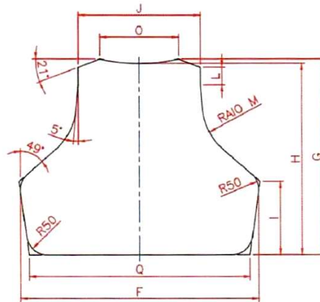
FIGURA 1 – Painéis Frontal e Dorsal, Modelo Estreito.
