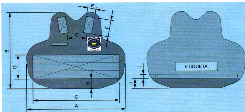
FIGURA 11 - Capa Frontal - Dimensionais
