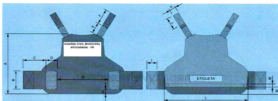
FIGURA 14 - Capa Dorsal - Dimensionais
