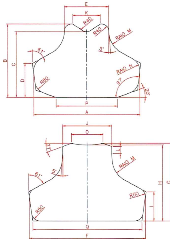
FIGURA 3 – Painéis Frontal e Dorsal, Modelo Largo.
