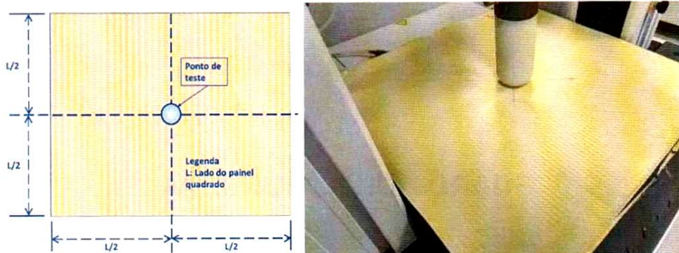
FIGURA 7 - Posicionamento do Painel Balístico Sobre a Plataforma do Teste de Flexibilidade.
