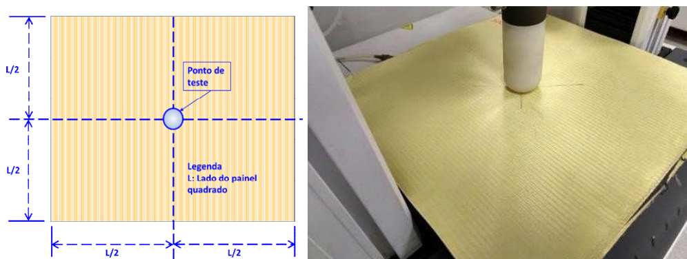
FIGURA 6 - POSICIONAMENTO DO PAINEL BALÍSTICO SOBRE A PLATAFORMA DO TESTE DE FLEXIBILIDADE.
