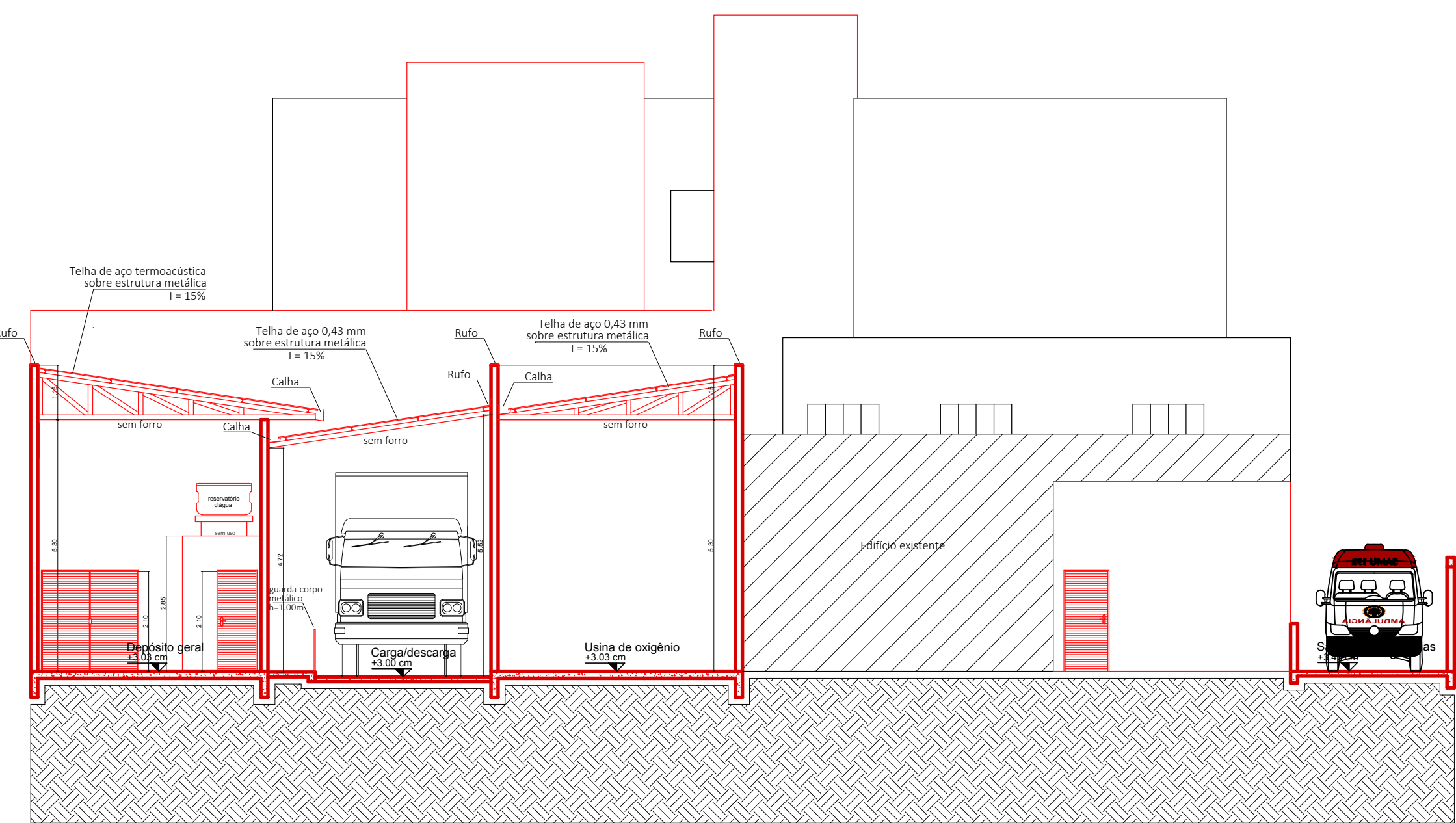
CORTE CC
