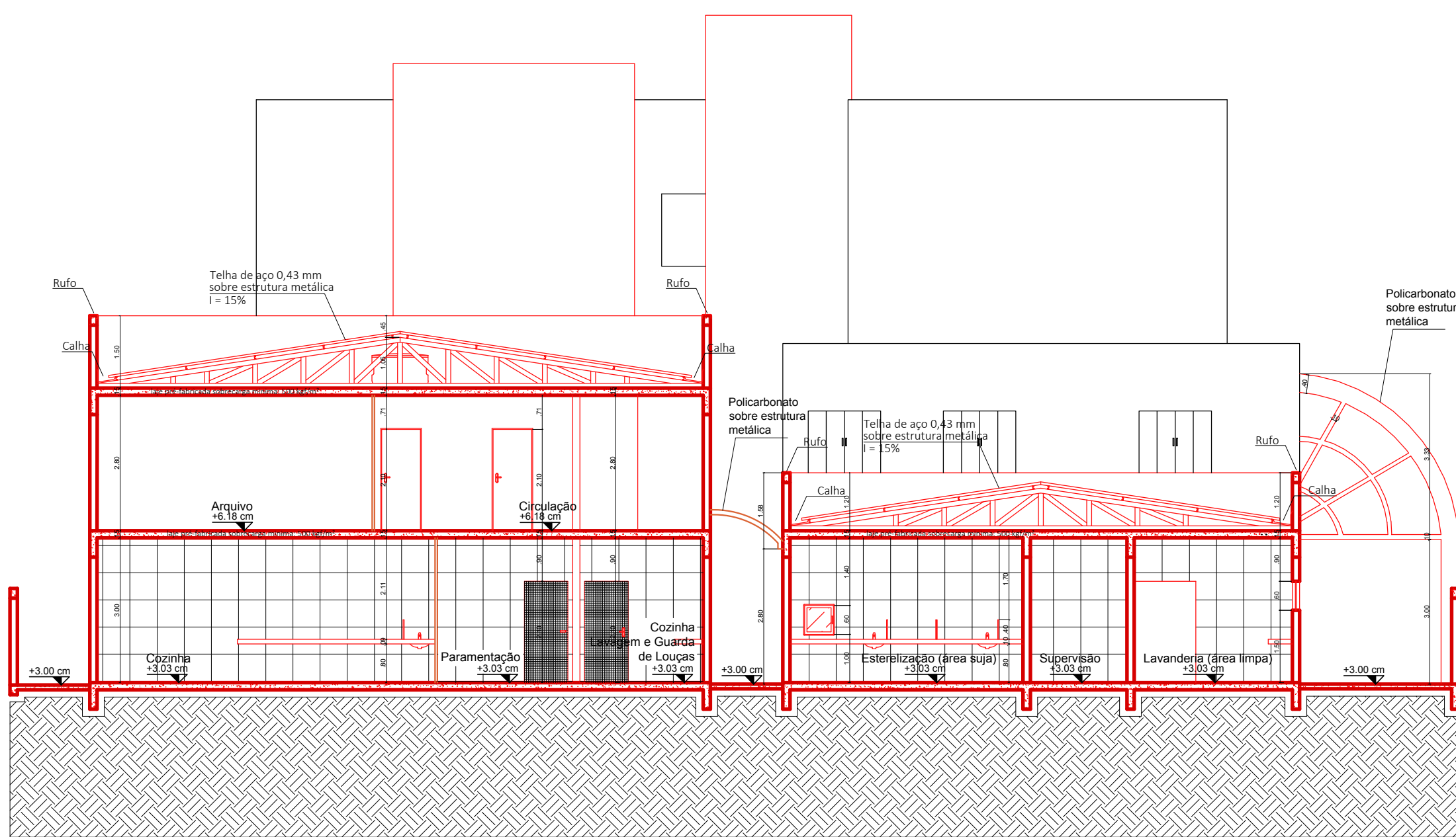
CORTE BB
